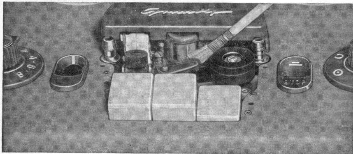
Abb. 6 Nach Abnahme der Drucktasten-Abdeckkappe sind die bandberührenden Teile des Tonbandgerätes für eine Säuberung gut zugänglich
