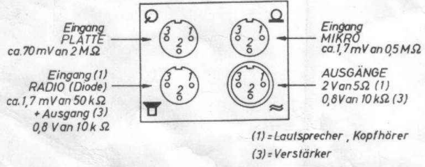
Blick auf die Anschlußbuchsen an der Kofferrückseite
